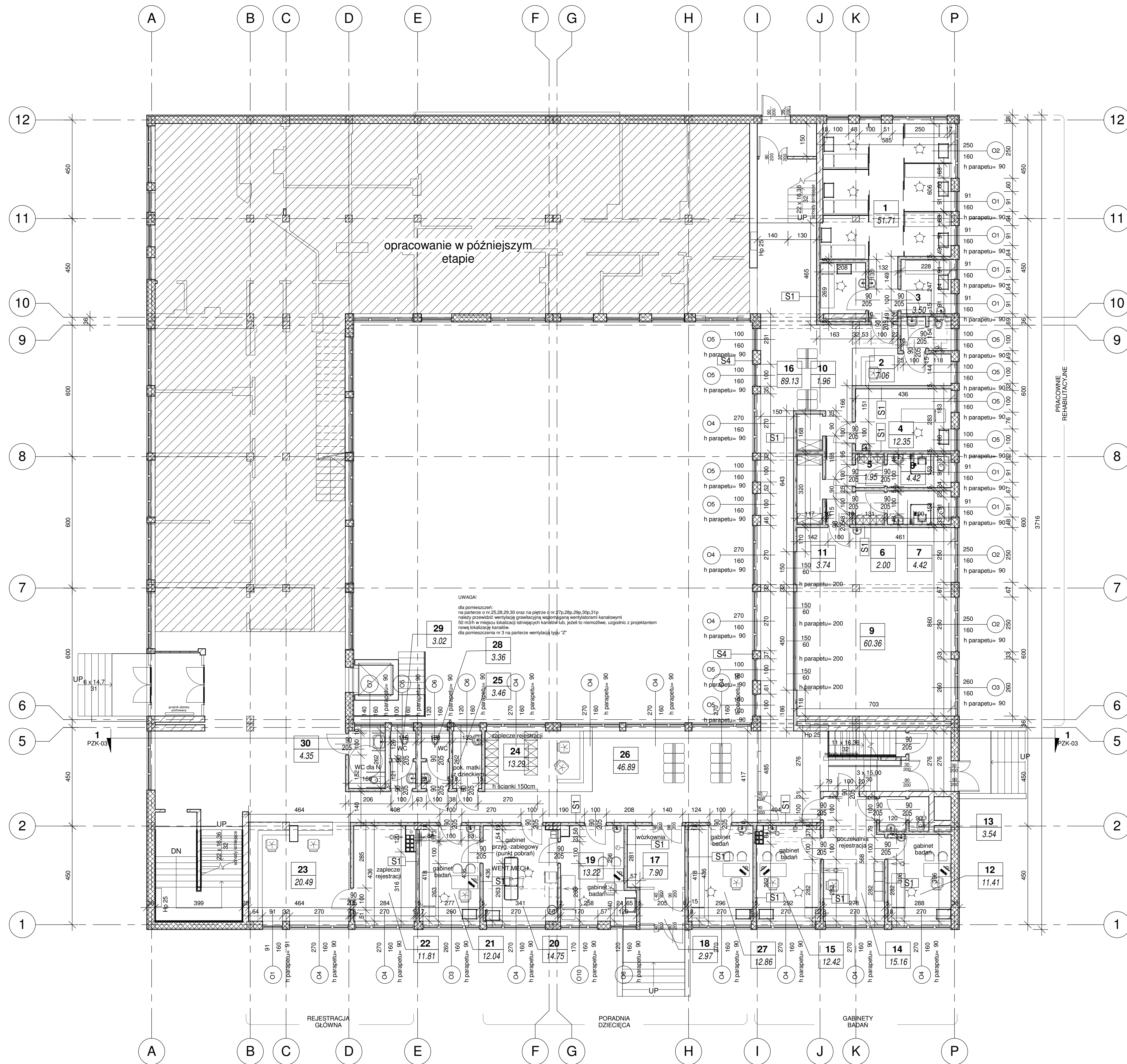
PARTER SKALA 1:100
